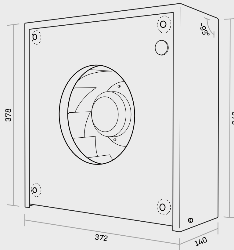
Måltegning af VK vægventilator (perspektiv)
