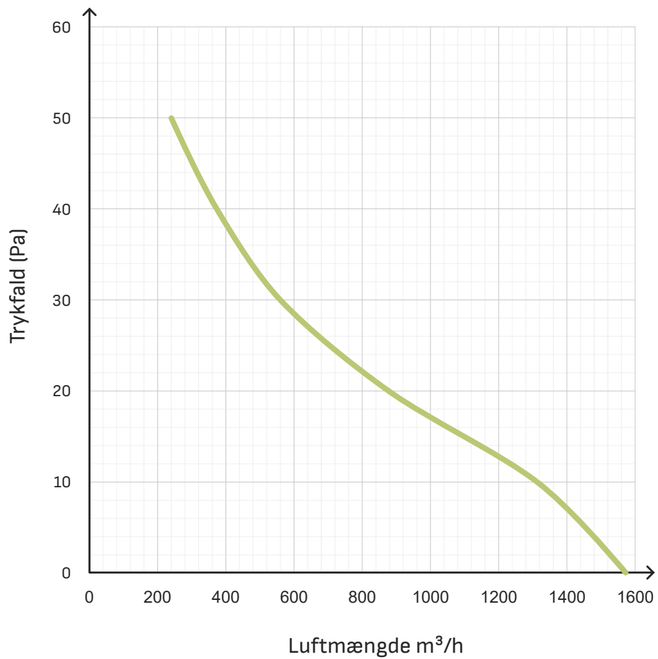
Kapacitetskurve
