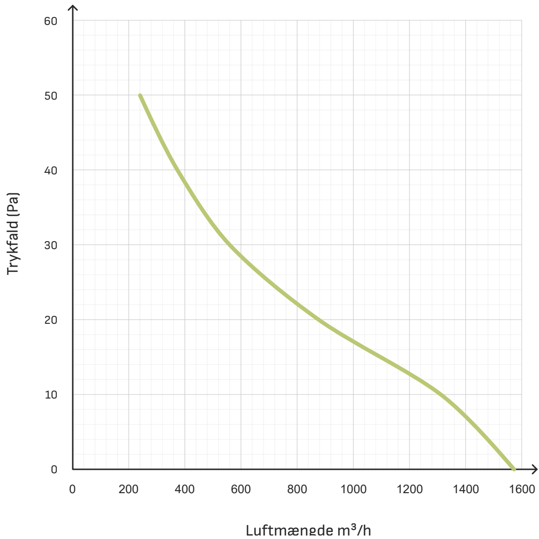
Kapacitetskurve
