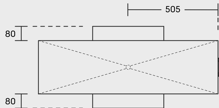
Plantegning: top
