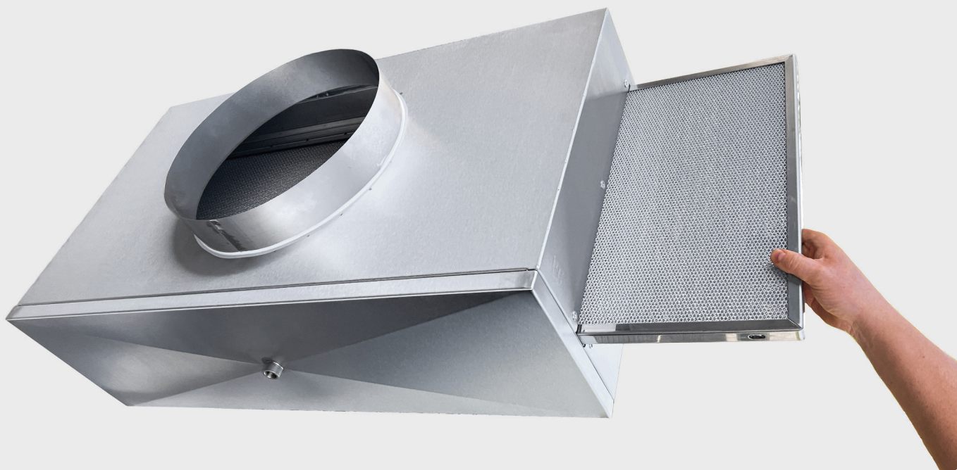
Åbent for-filter med udtagning af planfilter.
